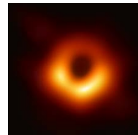
Erste veröffentlichte Darstellung des „Schattens“ und der Akkretionszuflüsse eines Schwarzen Lochs, berechnet aus Aufnahmen des Event-Horizon-Teleskops (Kern der Galaxie Messier 87)
